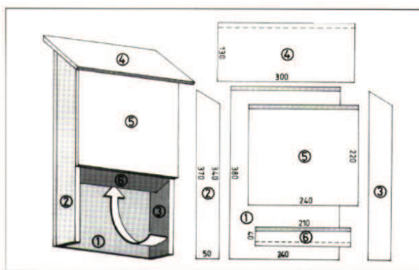
36 - Plan schématique du modèle Strassmann FS 1 (d'après Haensel et Nije 1982) - largeur de la fente d'accès entre (6) et (1) : 13 mm - inclinaison de la planchette (6) par rapport à la verticale : 60°
