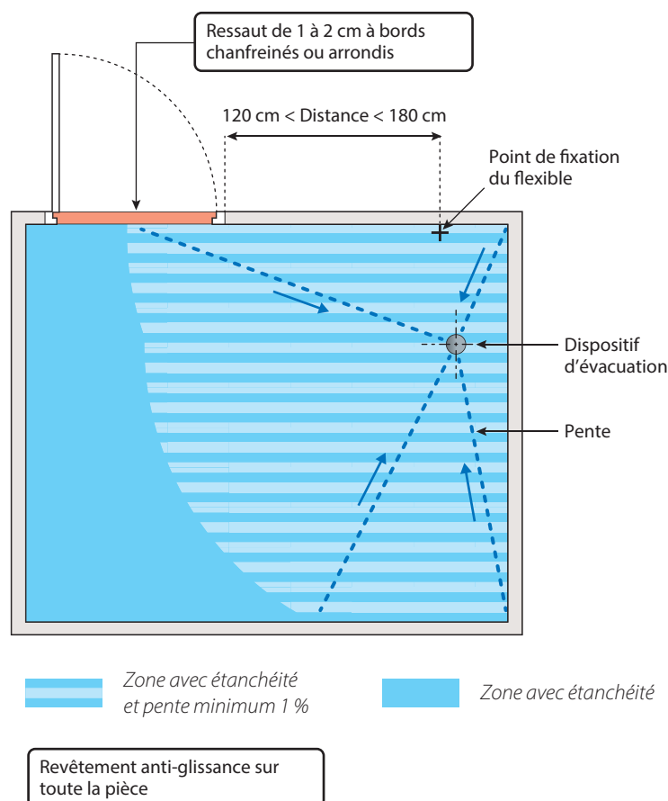
Figure 4 : Cas de la porte située dans la zone exposée à l'eau, c'est-à-dire entre 120 cm et 180 cm du point de fixation du flexible ou du dispositif d'évacuation
