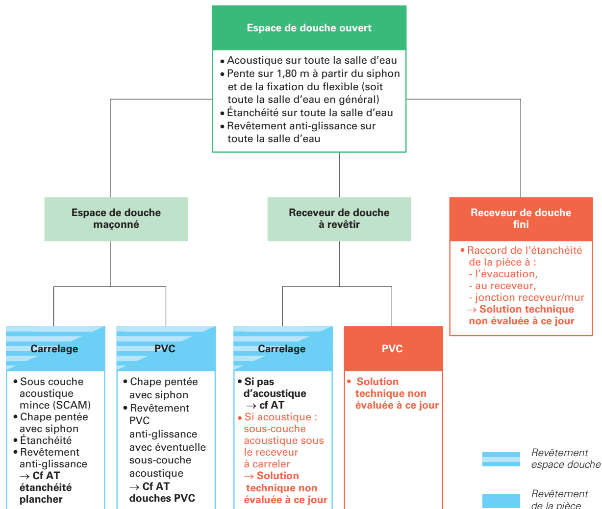
Figure 8 : Solutions de mise en œuvre pour les espaces de douche ouverts
