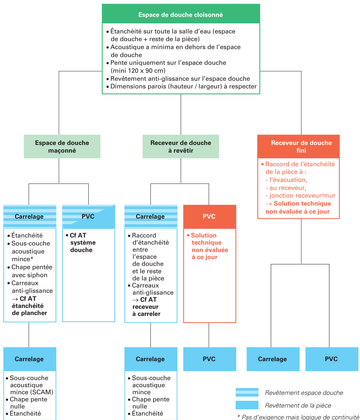
Figure 9 : Solutions de mise en œuvre pour les espaces de douche cloisonnés
