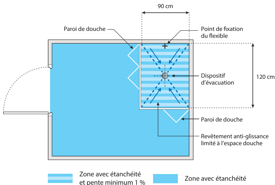
Figure 6 : Cas où les projections d'eau sont contenues
