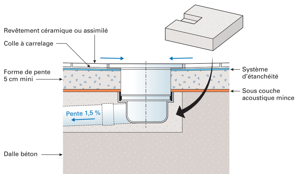
Figure 12 : Siphon encastré dans la dalle (saignée ponctuelle pour siphon et évacuation) (cas d'un revêtement de sol carrelé)
