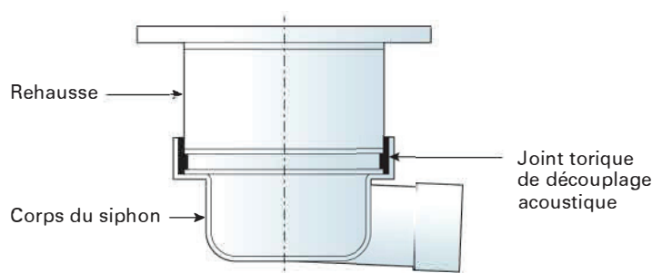
Figure 15 : Exemple de disposition permettant d'assurer un découplage entre la rehausse et le corps du siphon
