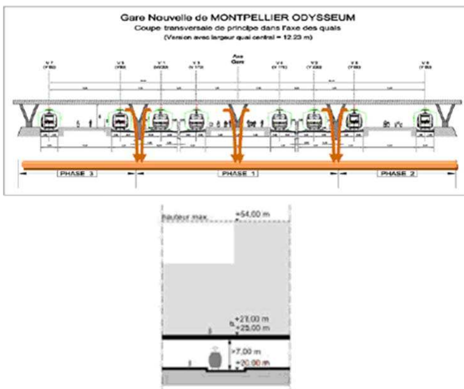
Figure 85 : Schéma d'insertion de la gare nouvelle
