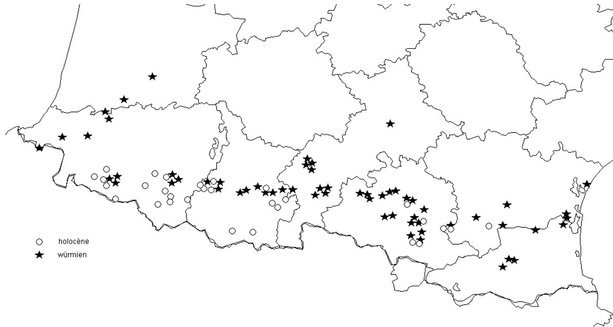
Figure 6 : localisation des gisements osseux de bouquetin au versant nord des Pyrénées
