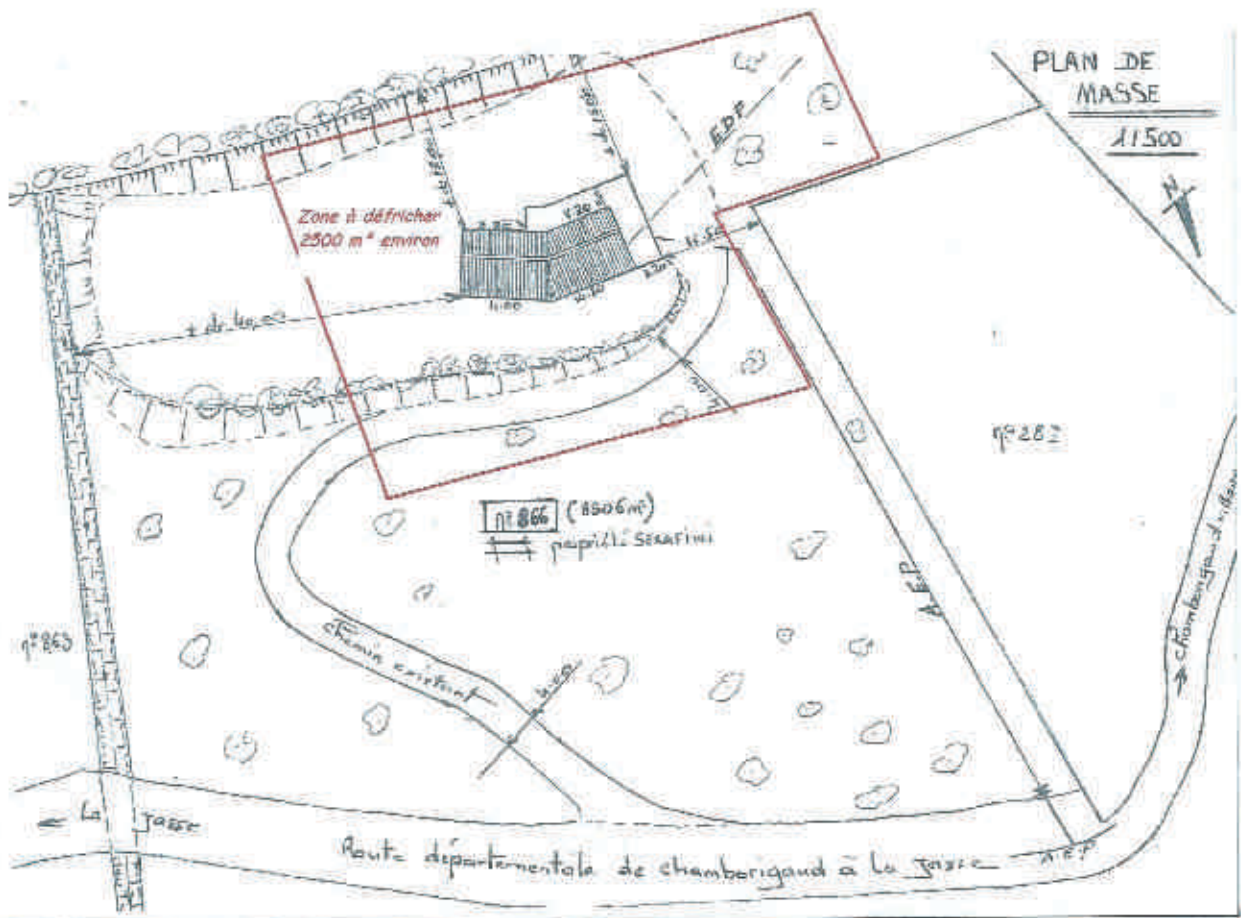
Plan de masse avec zone à défricher
