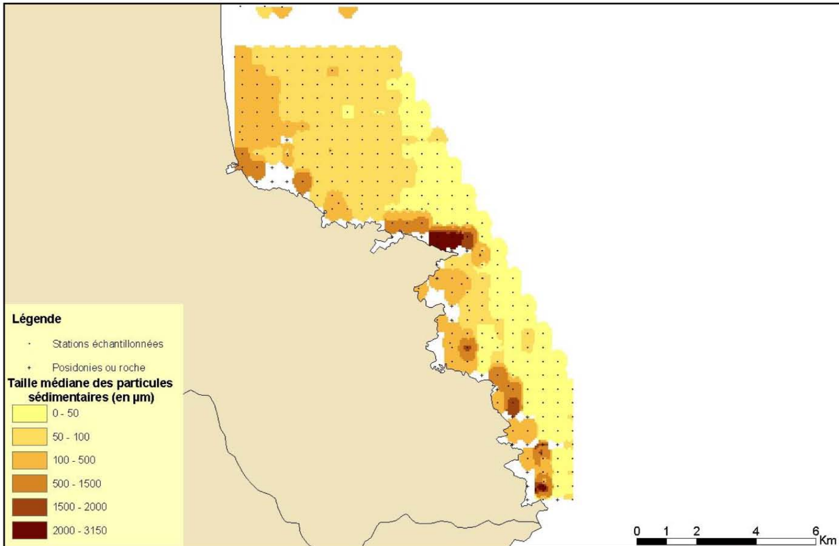
Carte 6. Granulométrie médiane de la zone échantillonnée (en µm)
