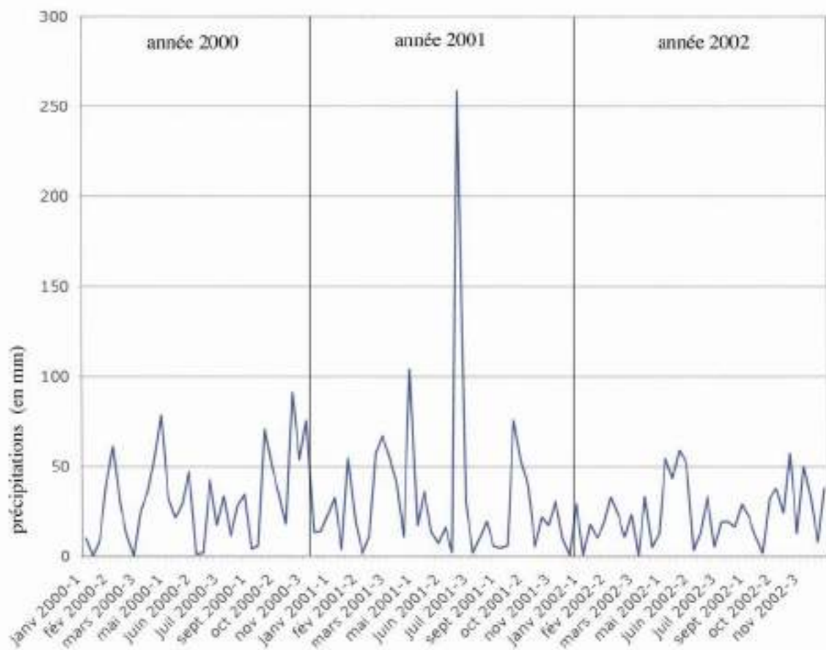
Fig. 1A. Pluviométrie par décade période 2000-2002 (station météo de Branceilles)
