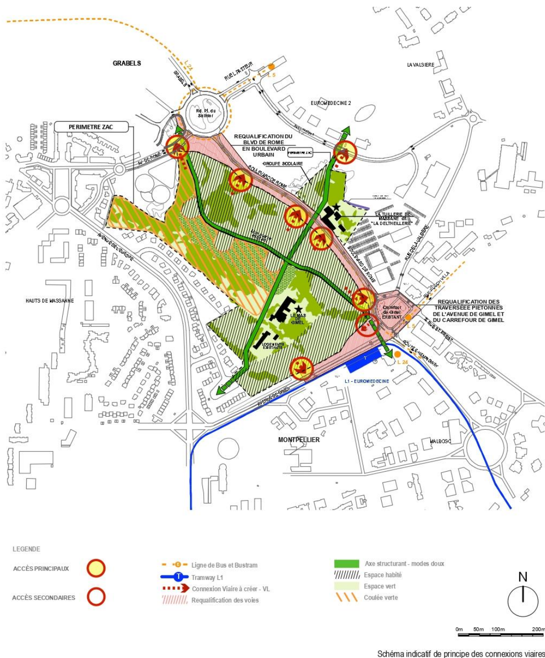
Figure 4 : schéma de principe indicatif des connexions viaires et accès
