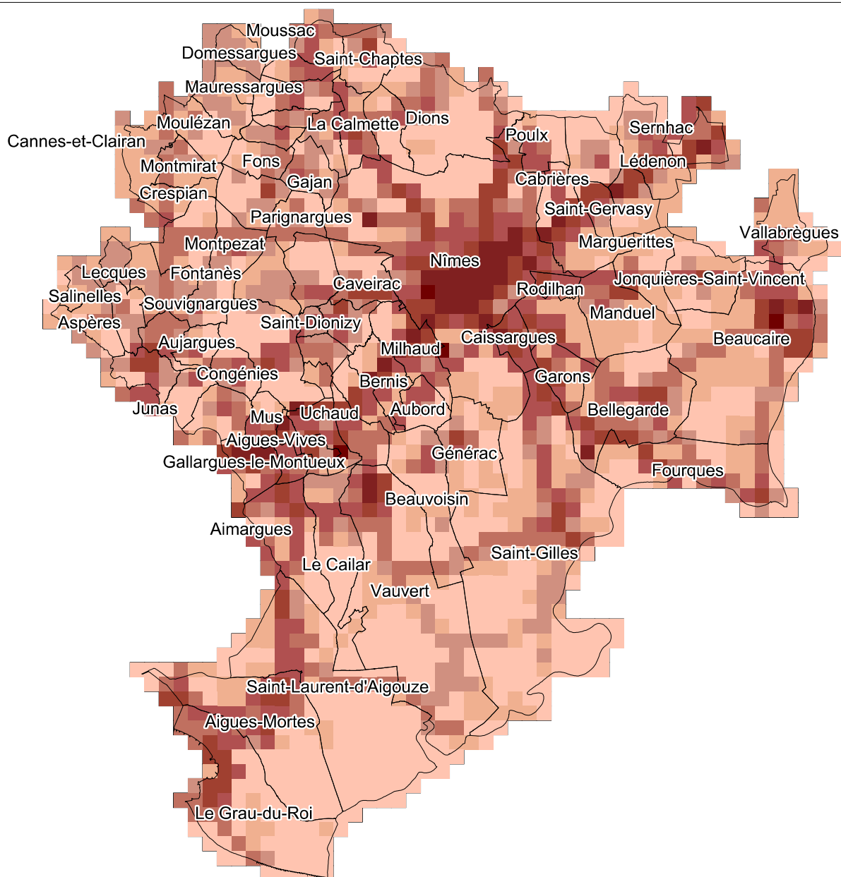
Emissions de CO 2 en t/km 2 /an
