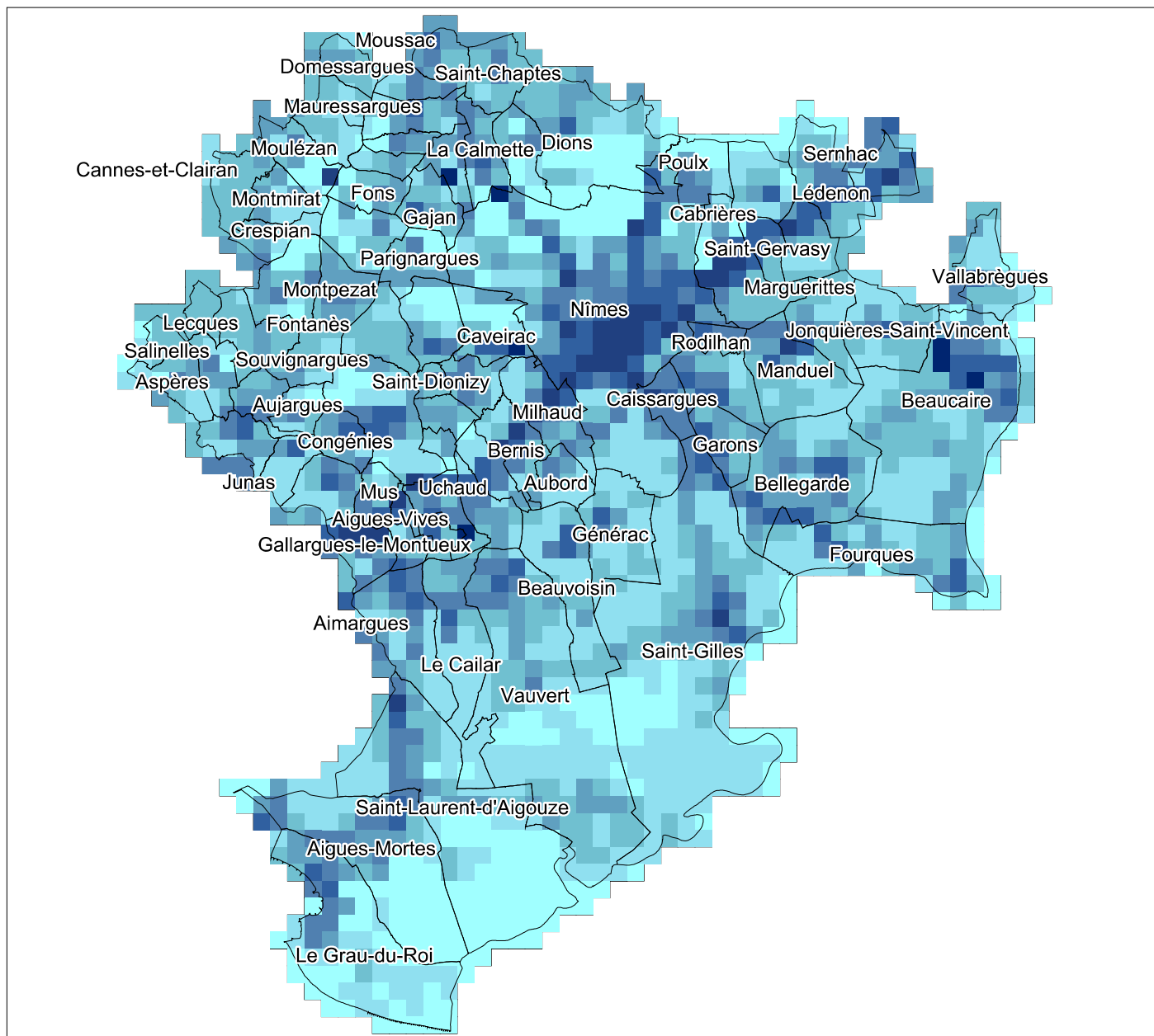
Emissions de PM 2,5 en kg/km 2 /an
