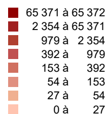
Emissions de SO 2 en kg/km 2 /an
