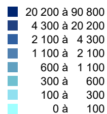
Emissions de PM10 en kg/km²/an
