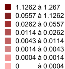
Emissions d'Arsenic en kg/km 2 /an
