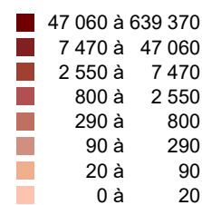
Emissions de CO 2 en t/km 2 /an
