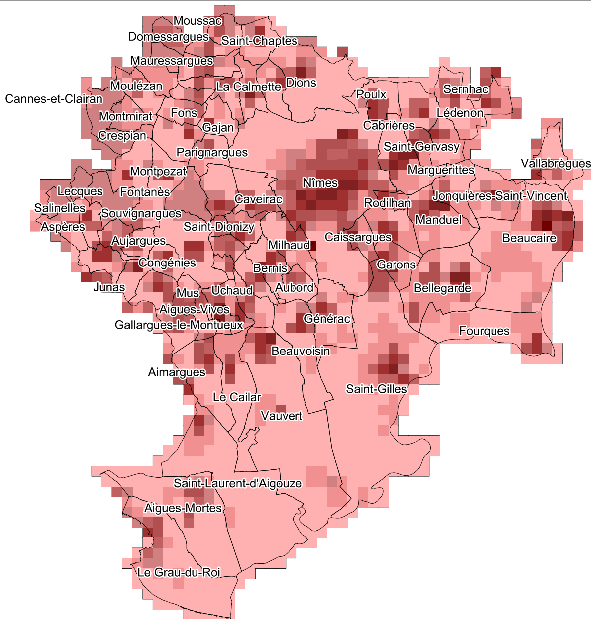
Emissions d'Arsenic en kg/km 2 /an
