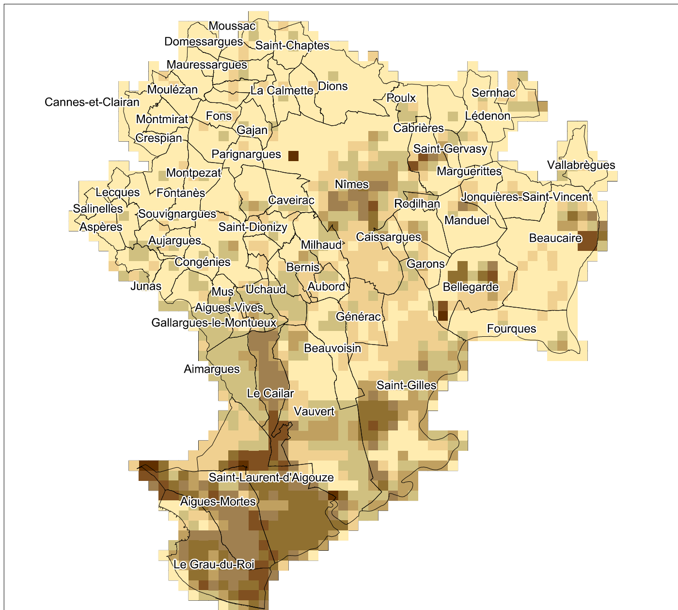
Emissions de CH 4 en t eq CO 2 /km 2 /an
