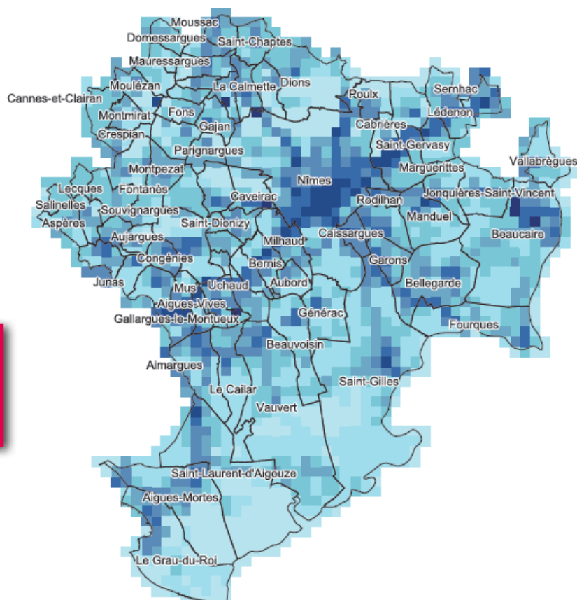
Figure 42 Localisation des émissions de PM 10 sur la zone PPA (kg/m 2 /an)
