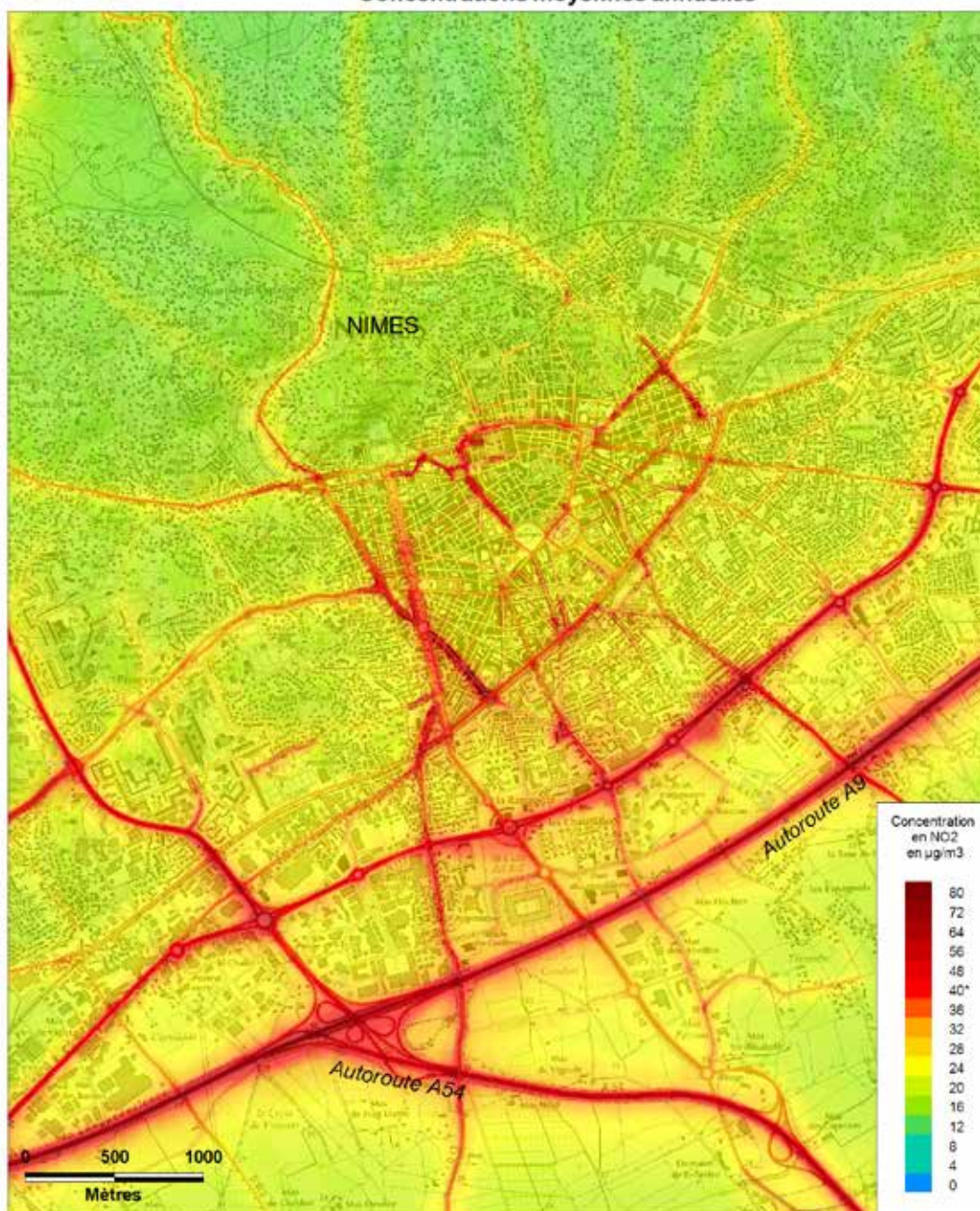
NO 2 - PPA de la zone urbaine de Nîmes - 2011 Etat initial Zoom ville de Nîmes Concentrations moyennes annuelles
