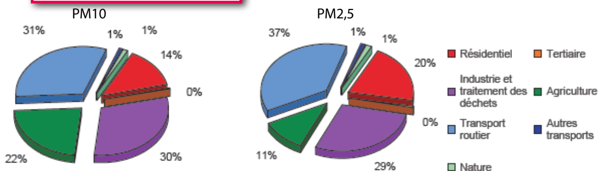
Figure 38 Répartition de l'origine des émissions de particules de la zone PPA– Année 2007
