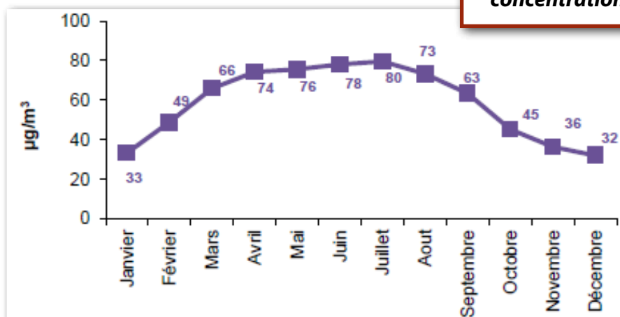
Figure 26 Profil moyen annuel des concentrations en ozone
