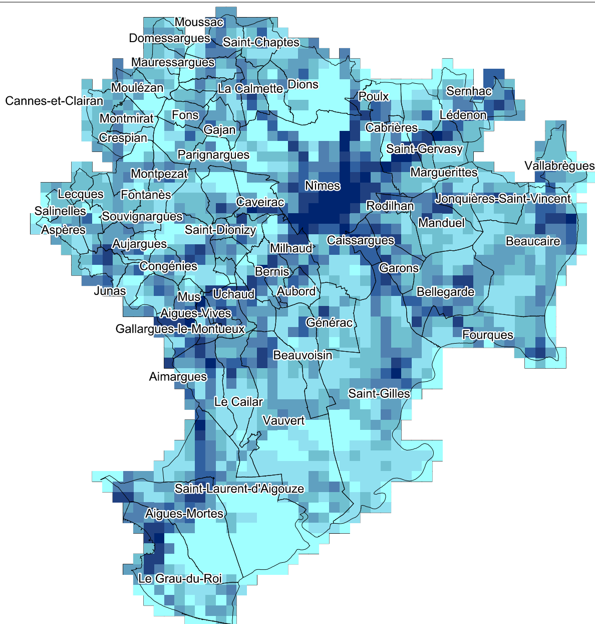
Part de chaque secteur dans les émissions de CO
