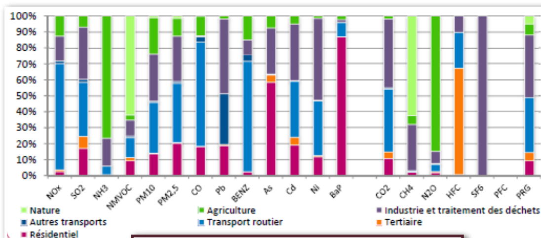
Figure 33 Répartition des secteurs d'activité à l'origine des émissions, année 2007 (source : AIR LR)
