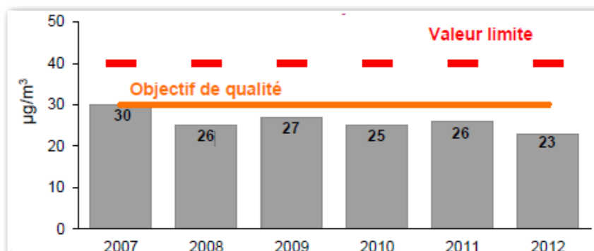
Milieu trafic routier - site de Nîmes-Gare
