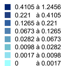
Emissions de BaP en kg/km 2 /an
