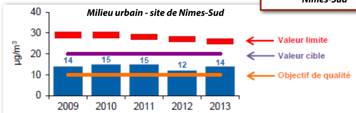
Figure 30 Moyennes annuelles en PM 2,5 au niveau du site Nîmes-Sud
