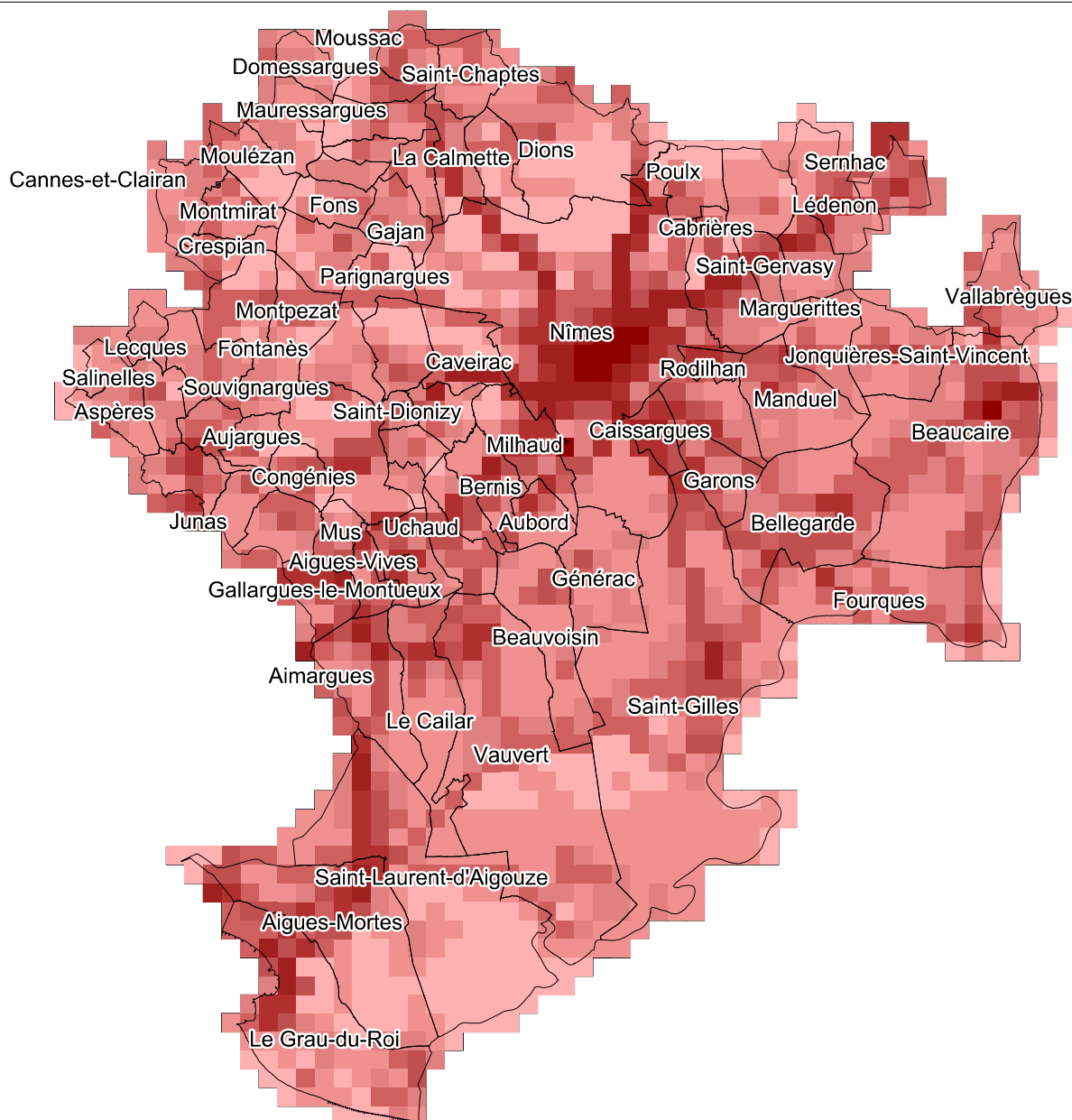
Part de chaque secteur dans les émissions de Benzène
