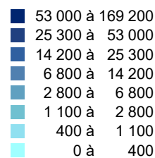
Emissions de CO en kg/km 2 /an
