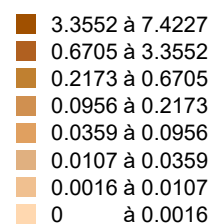
Emissions de Nickel en kg/km 2 /an
