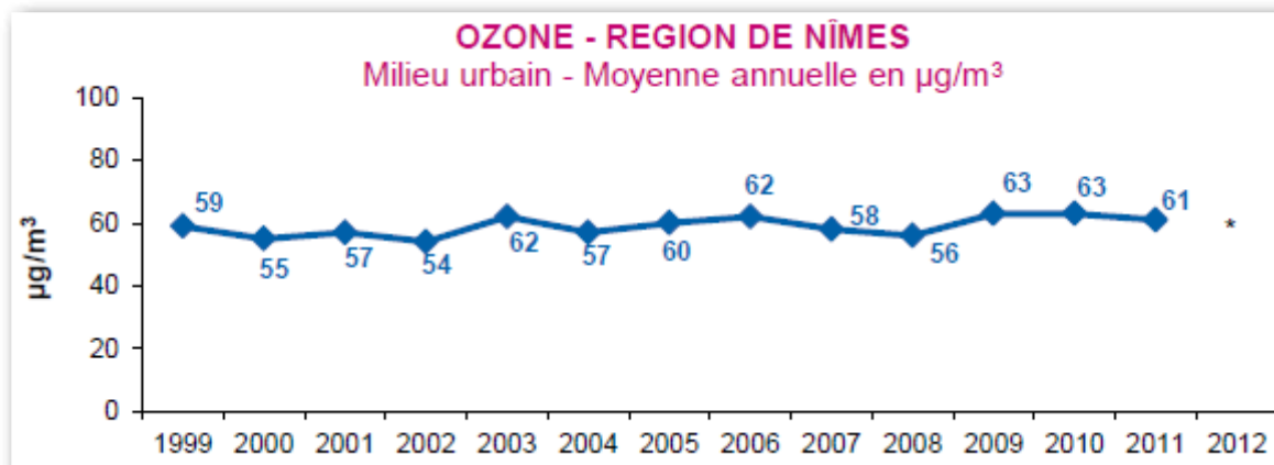
Figure 25 Évolution des concentrations annuelles moyennes en ozone dans la zone PPA
