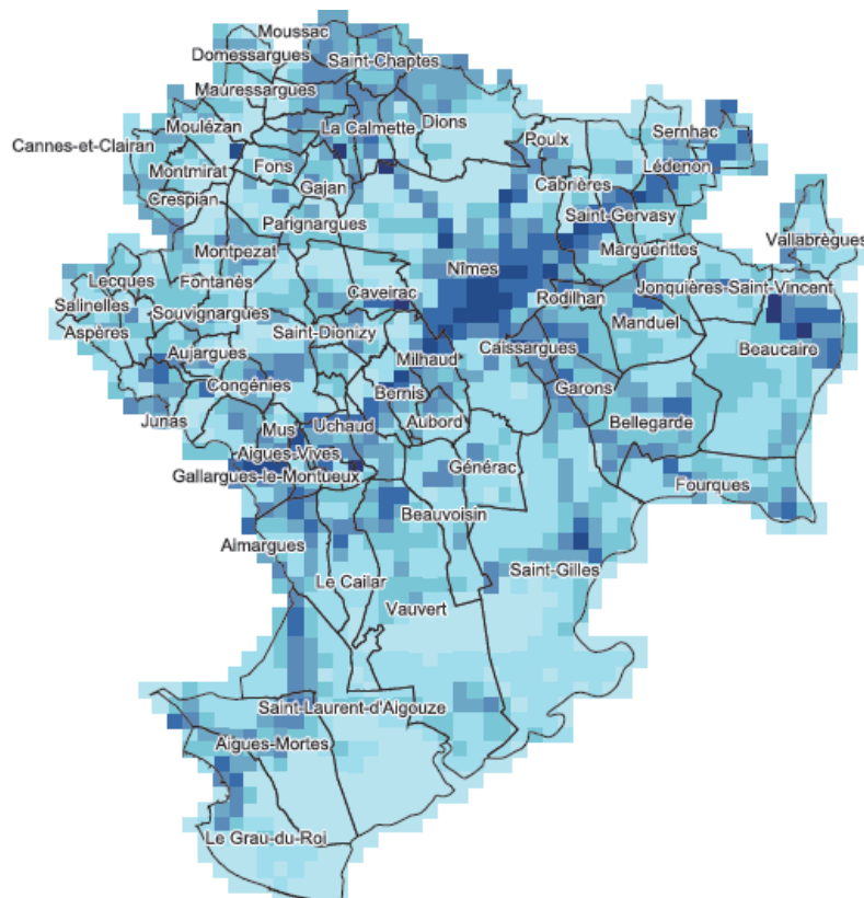
Figure 41 Localisation des émissions de PM 2,5 sur la zone PPA (kg/m 2 /an)
