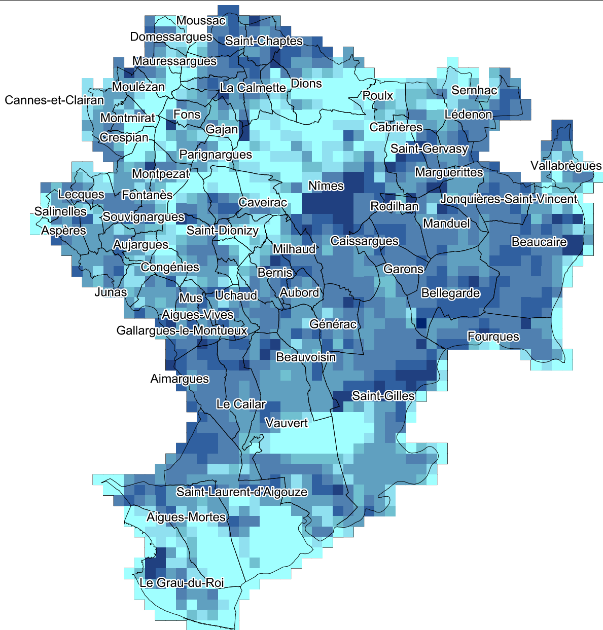
Part de chaque secteur dans les émissions de NH 3
