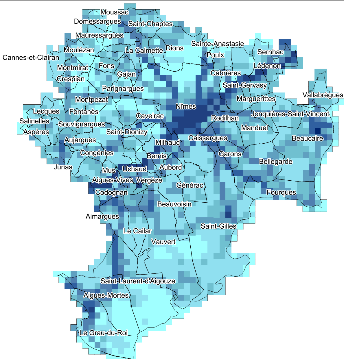
Part de chaque secteur dans les émissions de NOx
