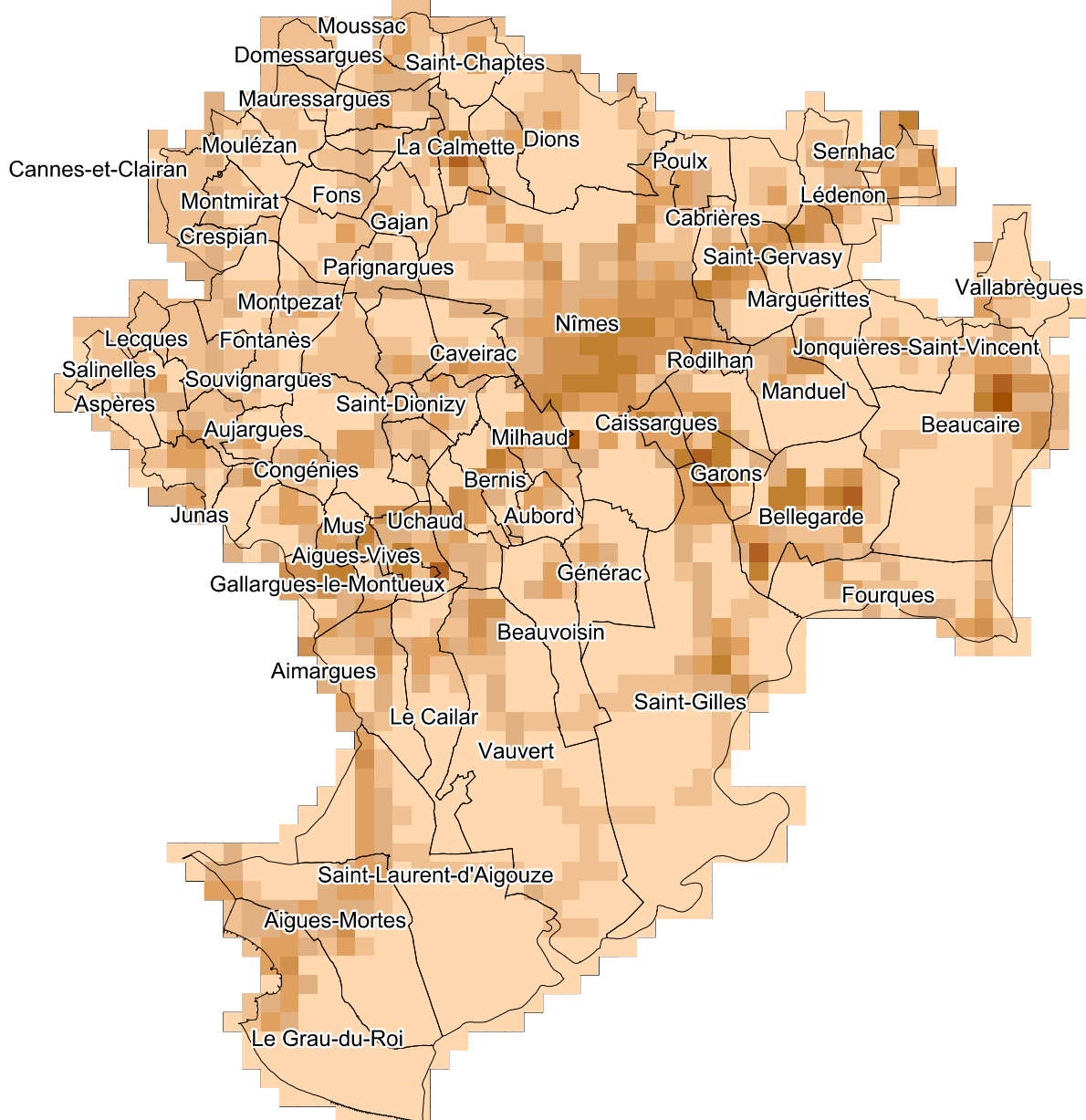
Part de chaque secteur dans les émissions de Nickel
