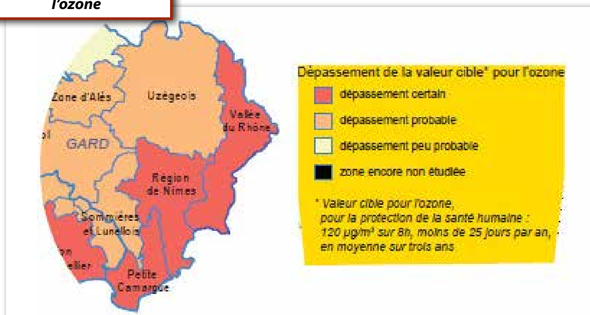
Figure 27 Évaluation des risques de dépassement pour l'ozone
