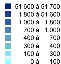
Emissions de NH 3 en kg/km 2 /an
