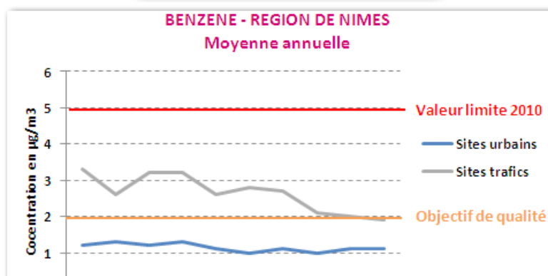
Figure 32 Concentrations moyennes annuelles en benzène entre 2001 et 2010
