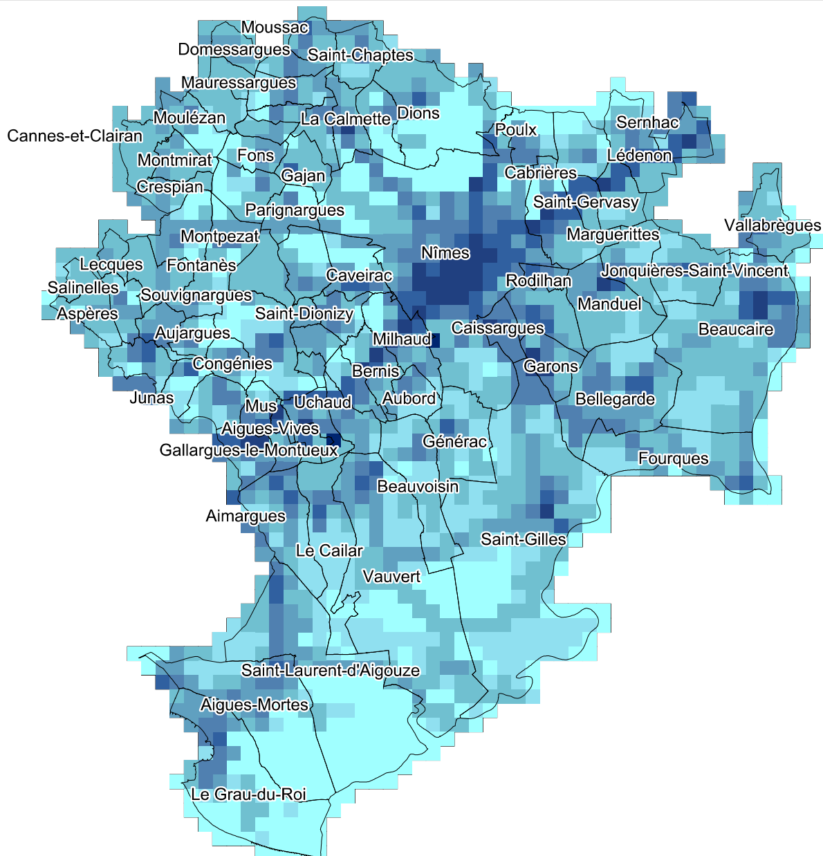
Emissions de Cadmium en kg/km 2 /an
