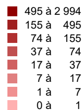
Emissions de Benzène en kg/km²/an
