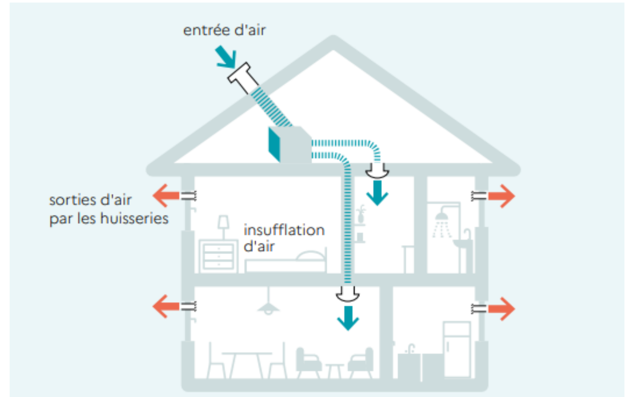
Schéma de principe VMI, source ADEME 1
