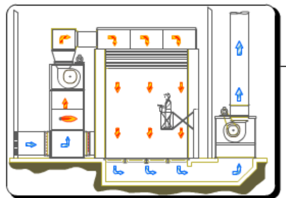
Cabine à ventilation verticale
