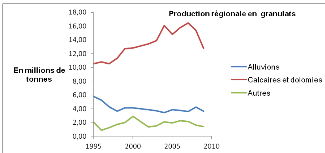
Figure 15 : Courbe de production en granulats issus de l'extraction de roches calcaires, de roches alluvionnaires et d'autres types de roches massives.
