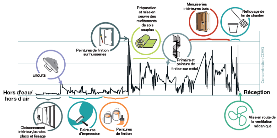
Évolution des concentrations en Composés Organiques Volatils Globaux
